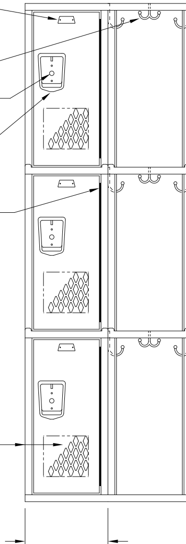
ELEVATION
