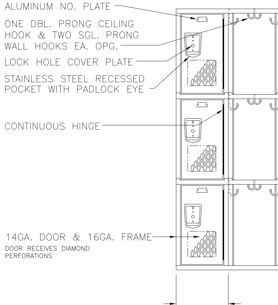
ELEVATION
