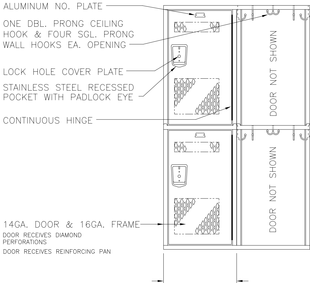
ELEVATION
